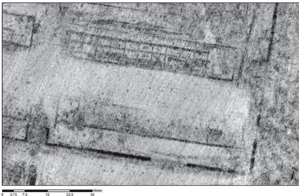
Fig. 8: Indagini georadar eseguite nel 2013 nella parte sud-est dell'area murata con profondità complessiva degli strati del sottosuolo di 50–100 cm (Istituto Ludwig Boltzmann per la Prospezione Archeologica e l'Archeologia Virtuale).
